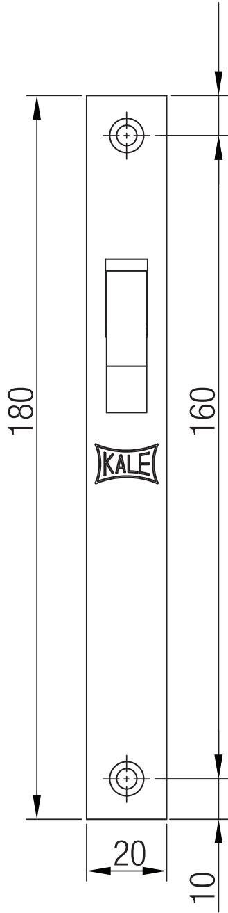
Açık Gövde Opened case
